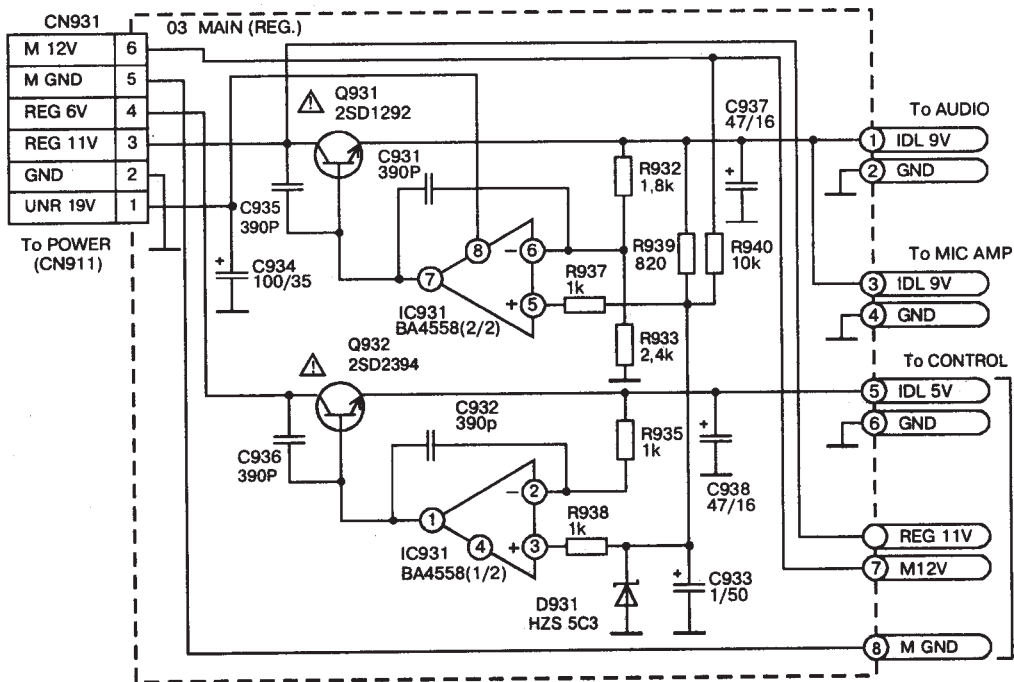
Принципиальная схема блока стабилизаторов напряжения видеомагнитофонов HR-P29A/78K.
